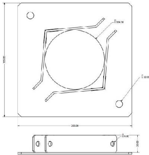
Klemmesystem 102
