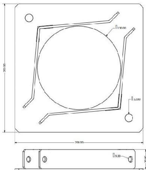
Klemmesystem 127
