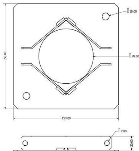
Klemmesystem 076
