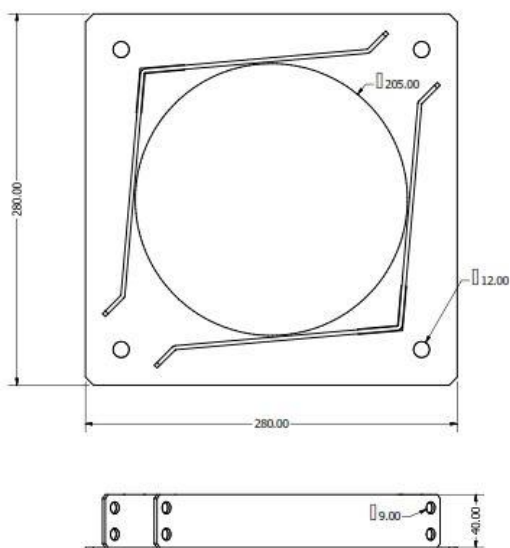
Klemmesystem 202
