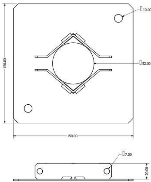
Klemmesystem 050
