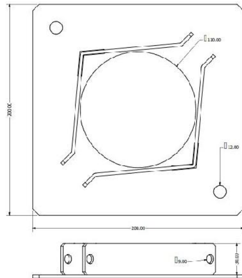
Klemmesystem 108
