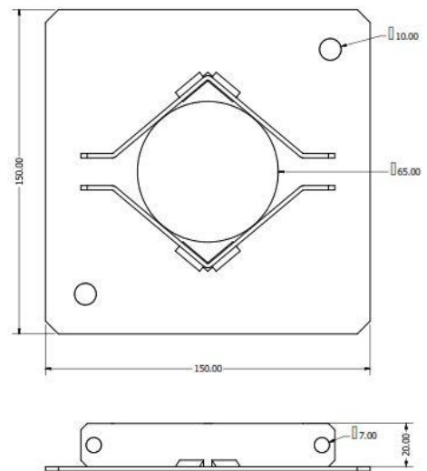
Klemmesystem 063
